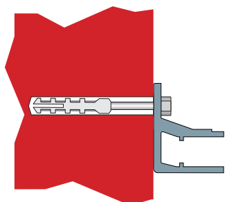
Монтаж в стена
